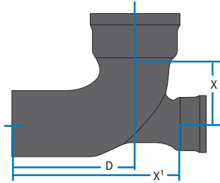
1/4 BEND w/ LOW HEEL INLET
